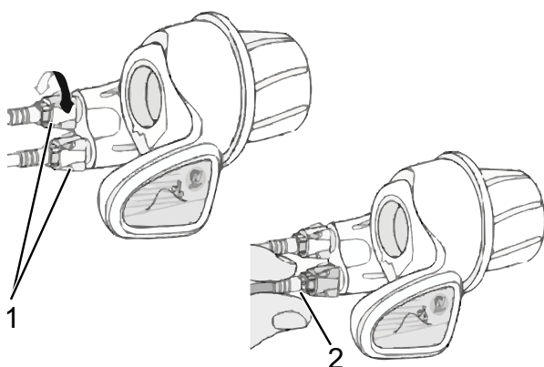
Figura 146: Interruttore a manopola del cambio con boccole di regolazione (1) e gioco della boccola del cambio (2)
