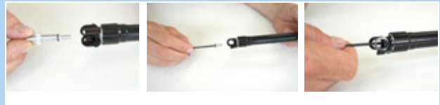
Figura 173: Fissaggio del coperchio della valvola della cartuccia
